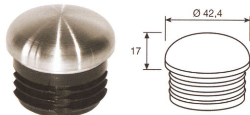
EX150 TAPPO BOMBATO Ø 42,4 - PLASTICA E ACCIAIO SATINATO
