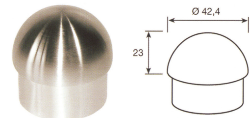
EX155 TAPPO BOMBATO Ø 42,4 - INOX AISI 304 SATINATO
