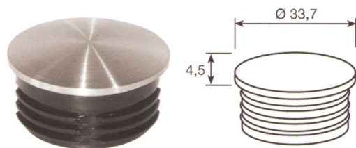
EX120 KIT TAPPO PIANO DN 33,7 PLASTICA E ACCIAIO SATINATO
