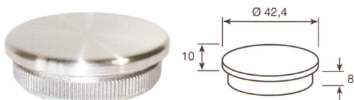
EX141 TAPPO PIANO Ø 42,4 - INOX AISI 304 SATINATO
