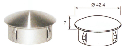
EX152 TAPPO LEGGERO Ø 42,4 - INOX AISI 304 SATINATO
