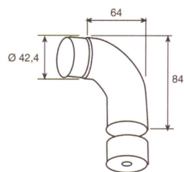
EX166 CURVA Ø 42,4 CON TAPPO FILETTATO - INOX AISI 304 SATINATO
