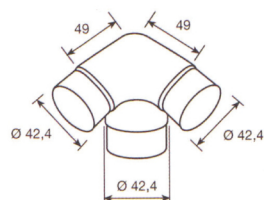
EX190 ANGOLO A TRE VIE Ø 42,4 - INOX AISI 304 SATINATO
