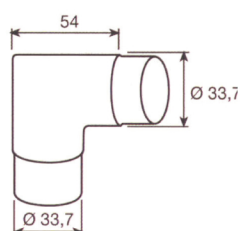
EX171 ANGOLO Ø 33,7 - INOX AISI 304 SATINATO
