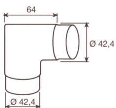
EX170 ANGOLO Ø 42,4 - INOX AISI 304 SATINATO
