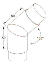
EX175 ANGOLO A 45° Ø 42,4 - INOX AISI 304 SATINATO
