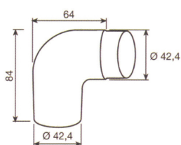
EX165 CURVA Ø 42,4 MASCHIO/FEMMINA - INOX AISI 304 SATINATO
